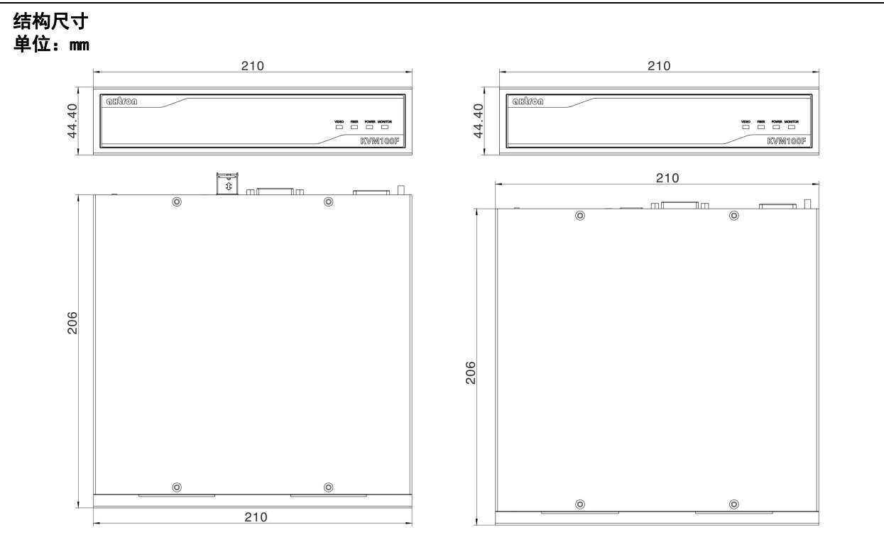
发射机（TX）、接收机（RX）正面视图
